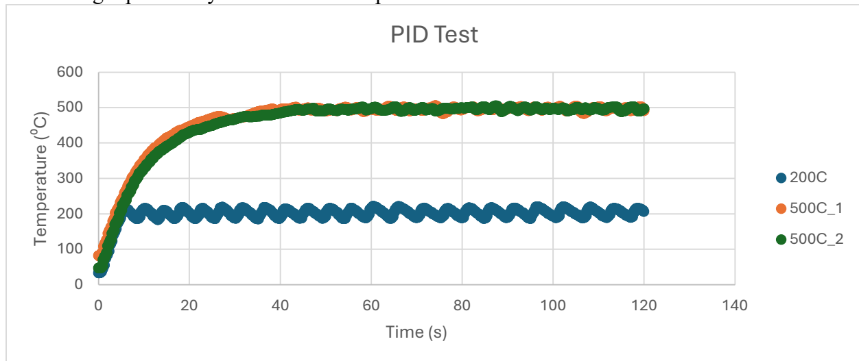
Figure 16: PID Set Point Test, Maiorov 2026
