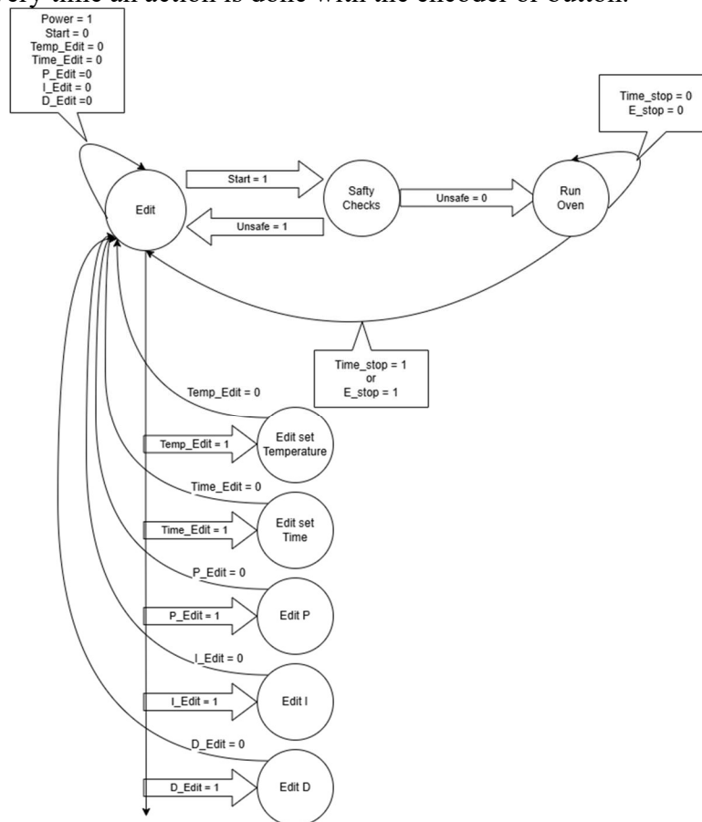
Figure 4: Logic Diagram, Maiores 2026
