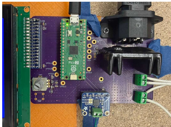
Figure 18: Final PCB, Maiorov 2026
